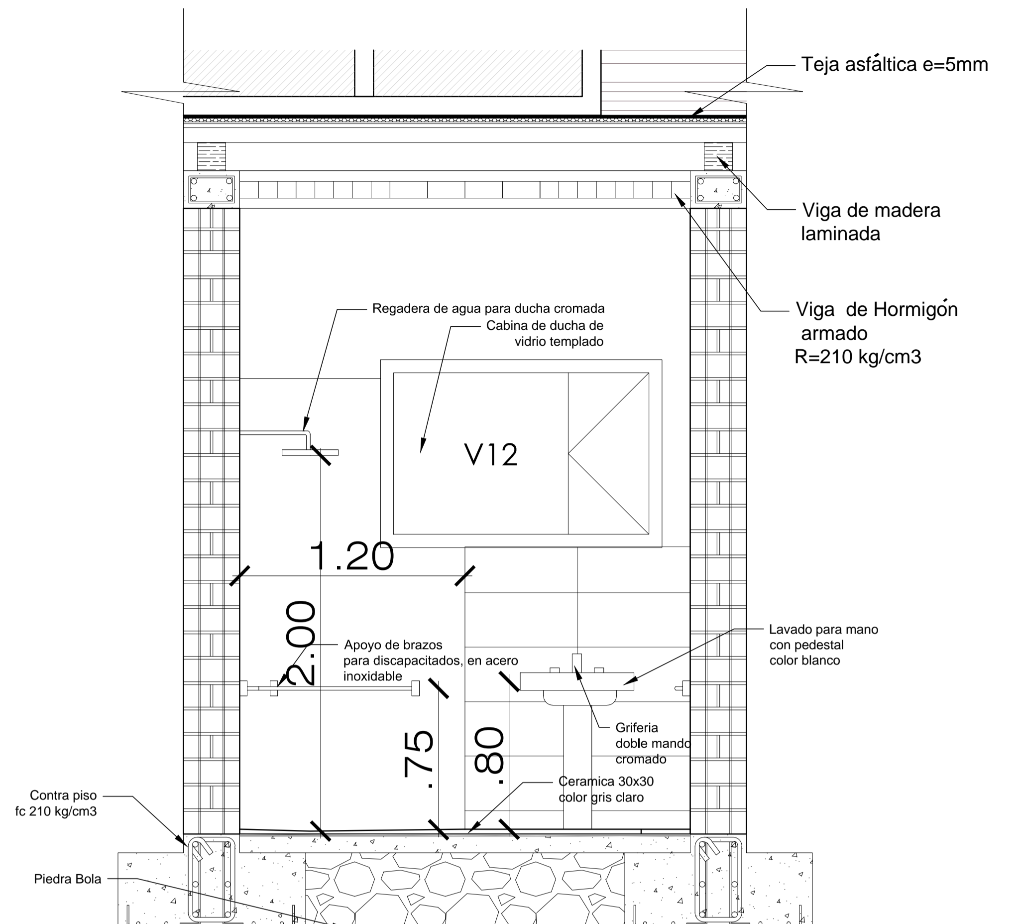
CORTE D D' Esc 1:25
