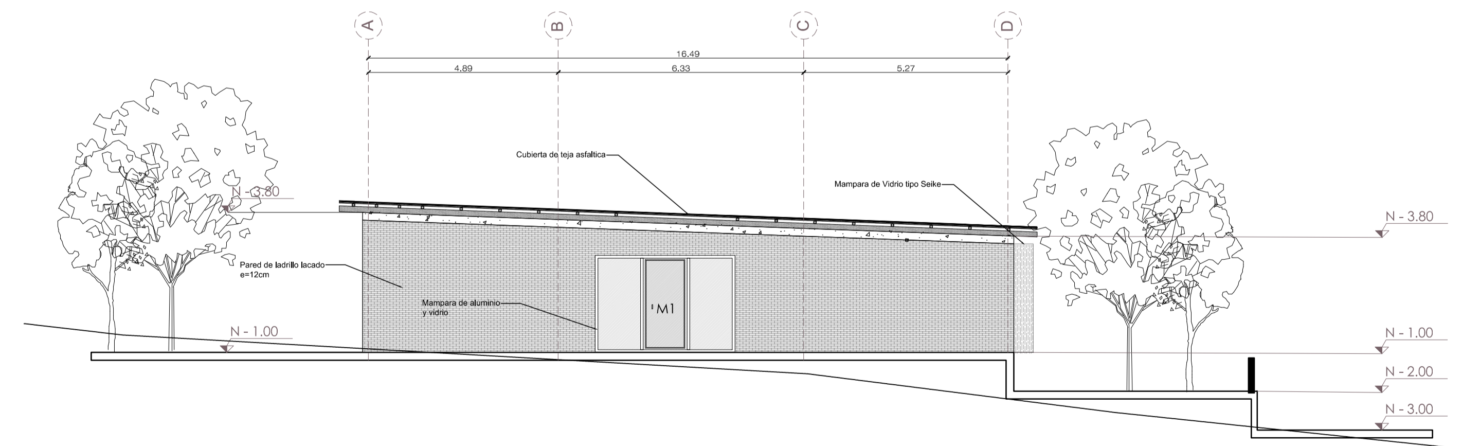
FACHADA LATERAL DERECHA
