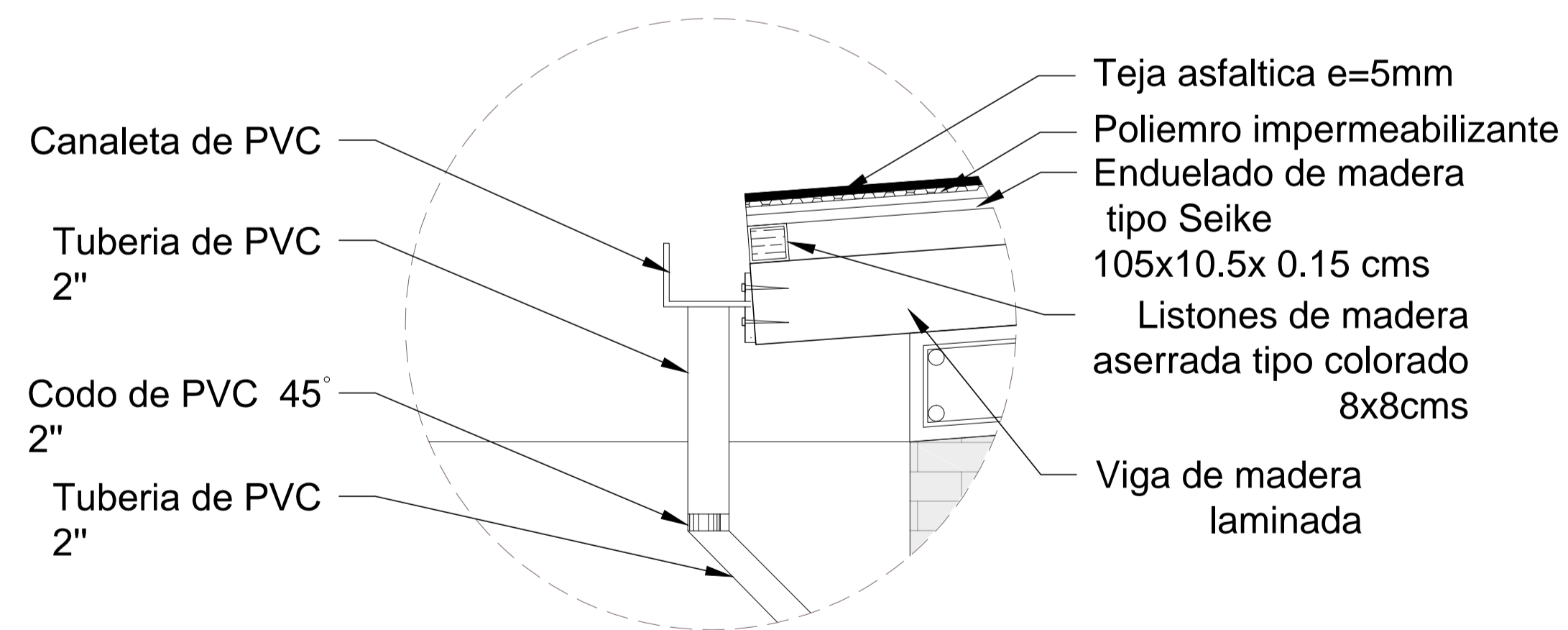
Esc 1:10 DETALLE CONSTRUCTIVO DC3
