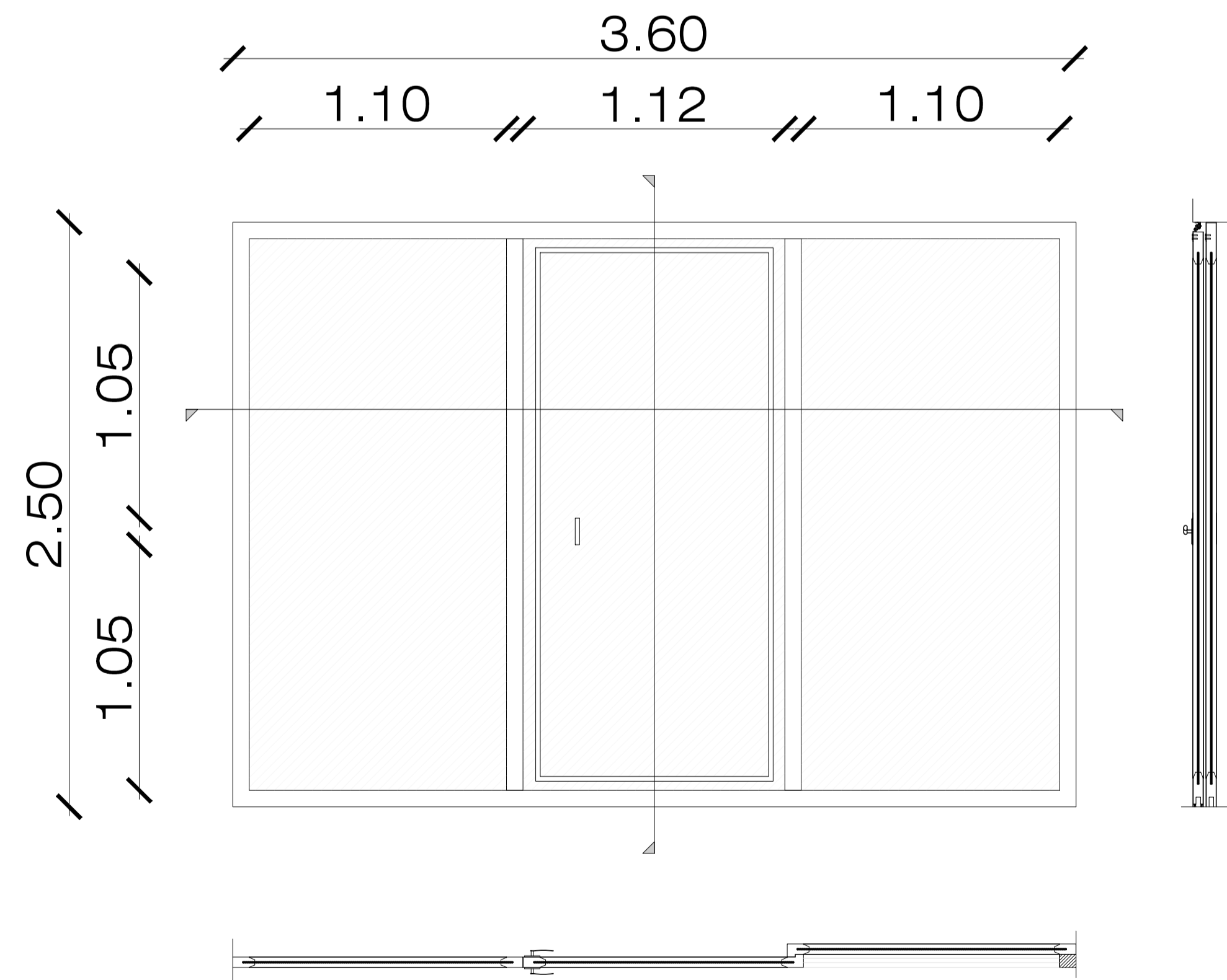
DETALLE DE PUERTA DE VIDRIO Esc 1:20
