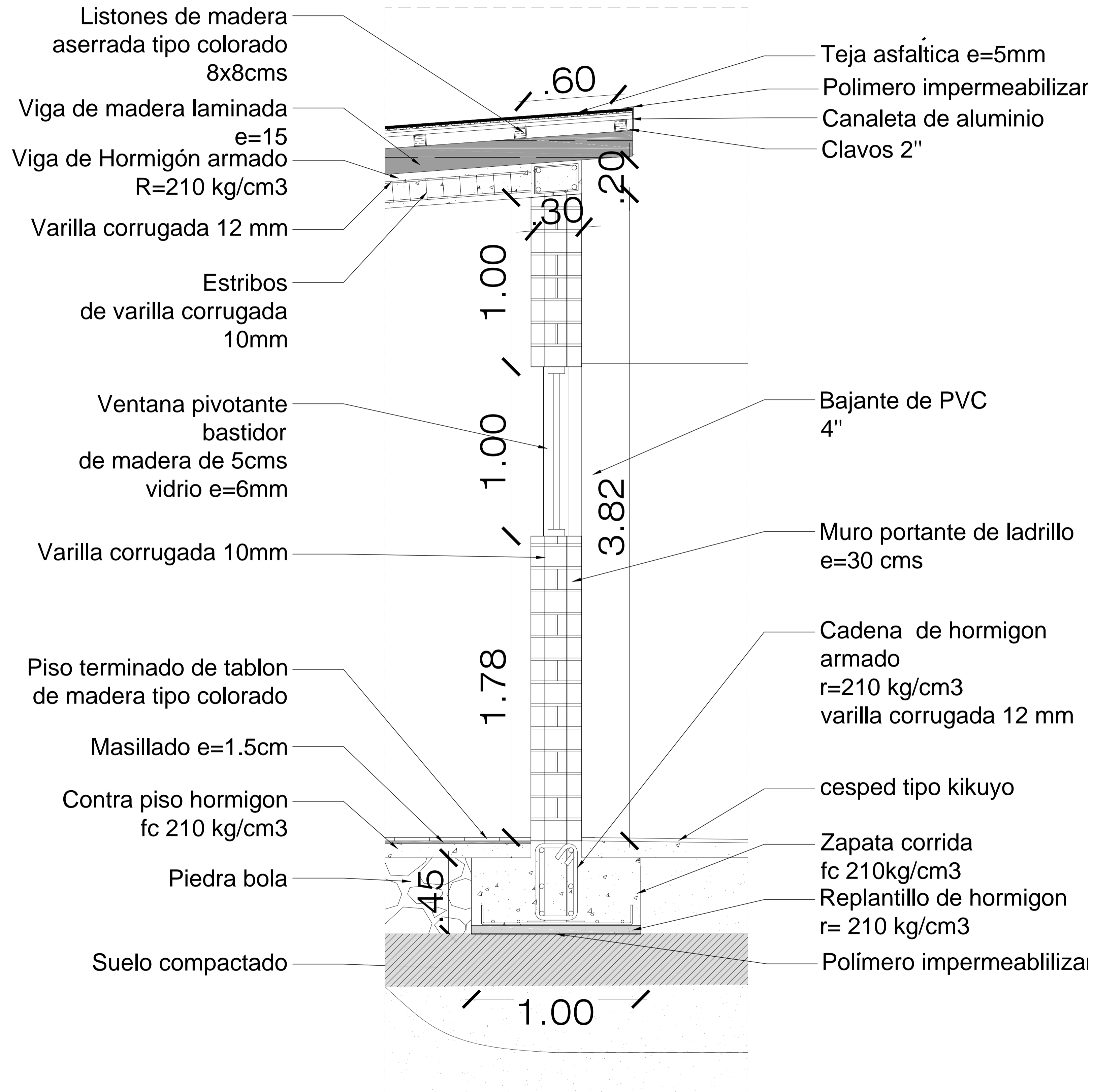
CORTE POR MURO Esc 1:15
