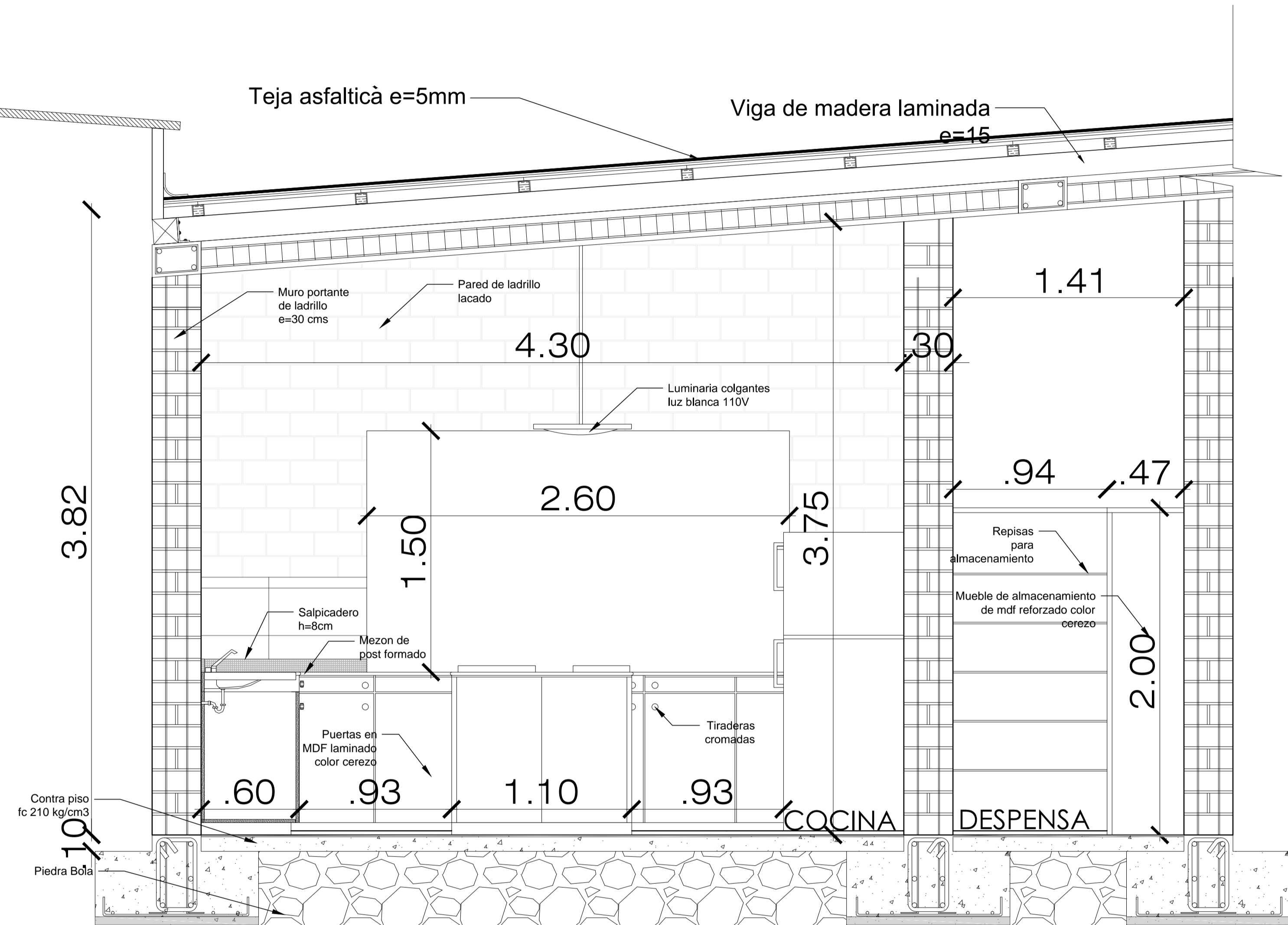
CORTE D-D' Esc 1:750
