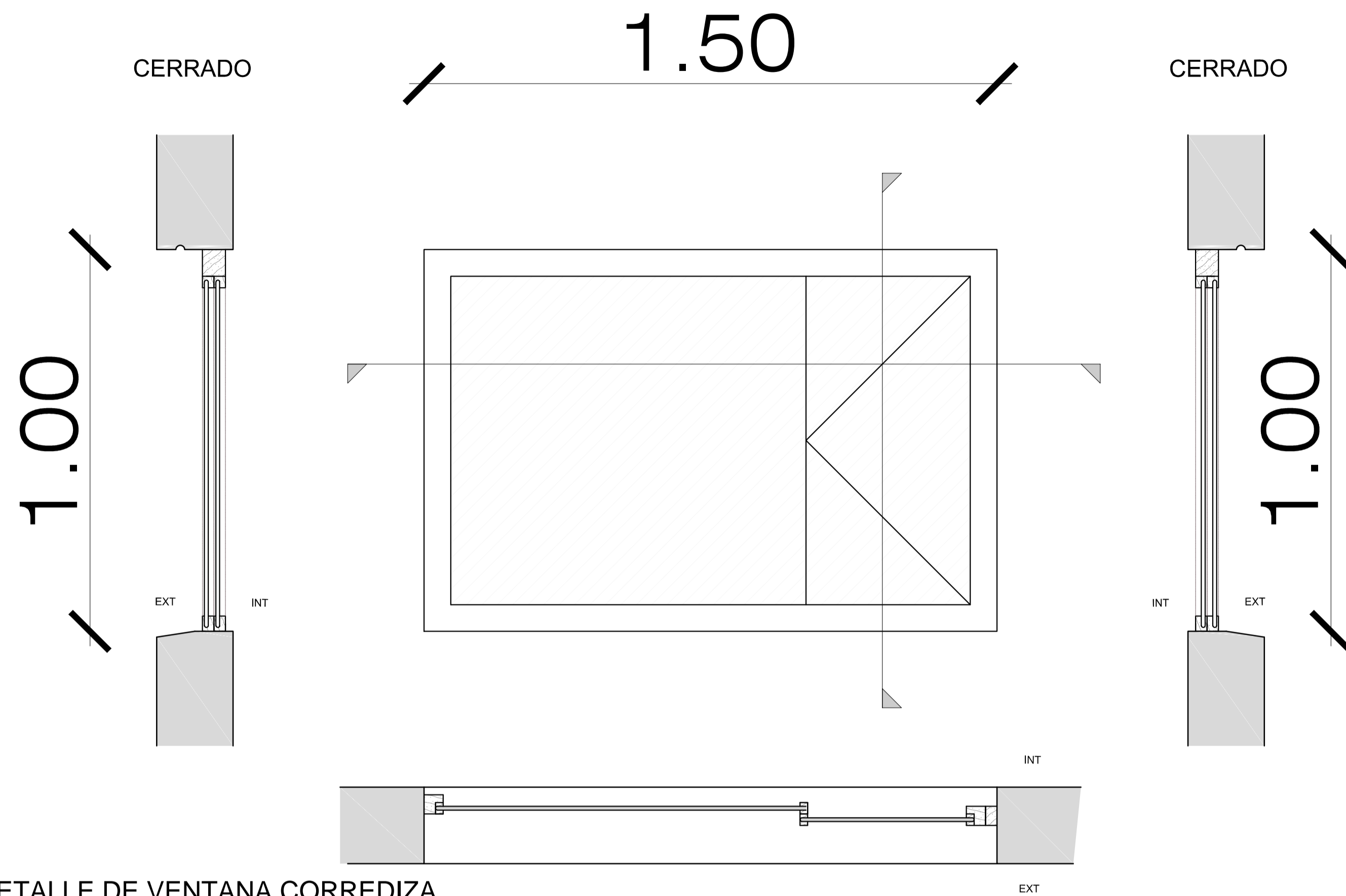
DETALLE DE VENTANA CORREDIZA Esc 1:10
