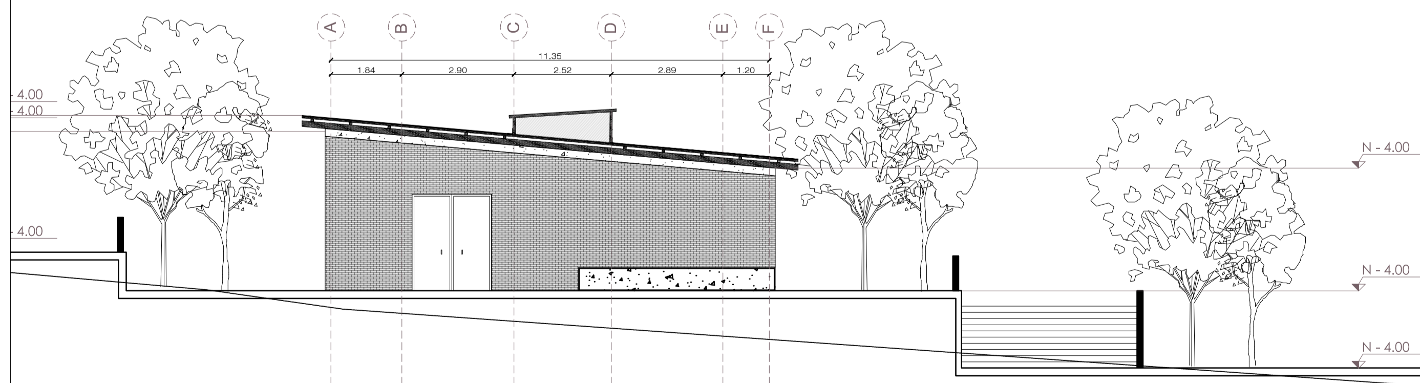
FACHADA LATERAL IZQUIERDA
