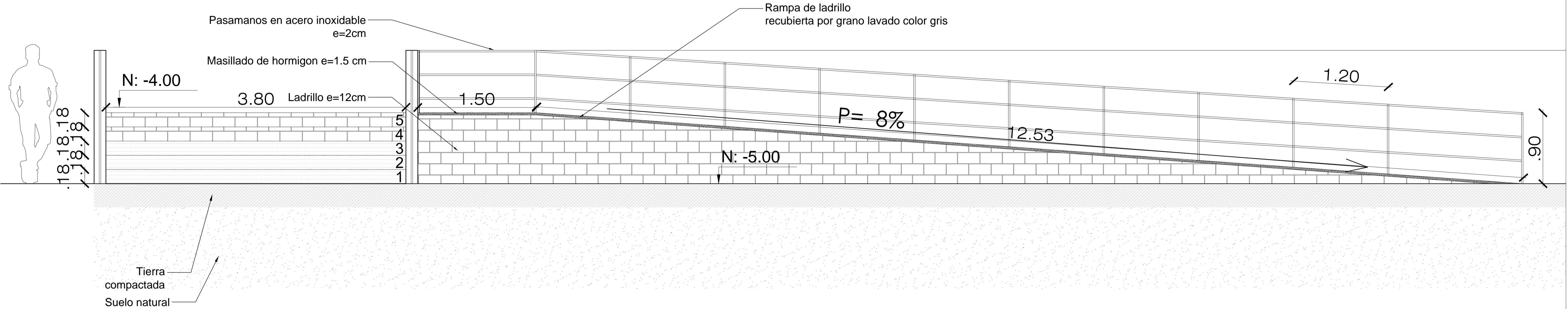
CORTE A - A' Esc 1:25
