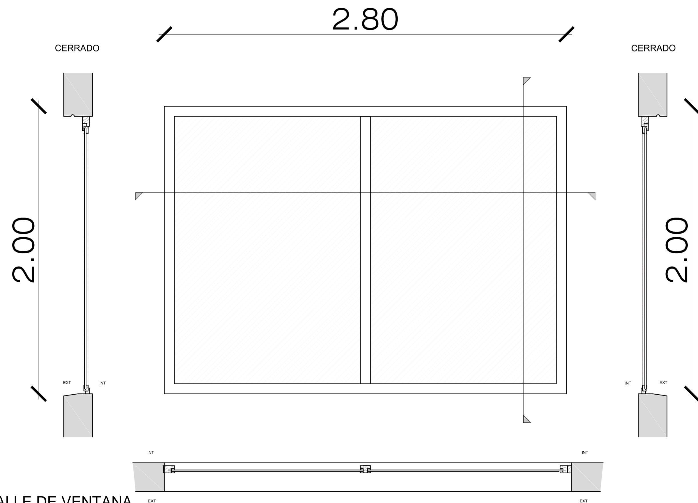
DETALLE DE VENTANA Esc 1:10
