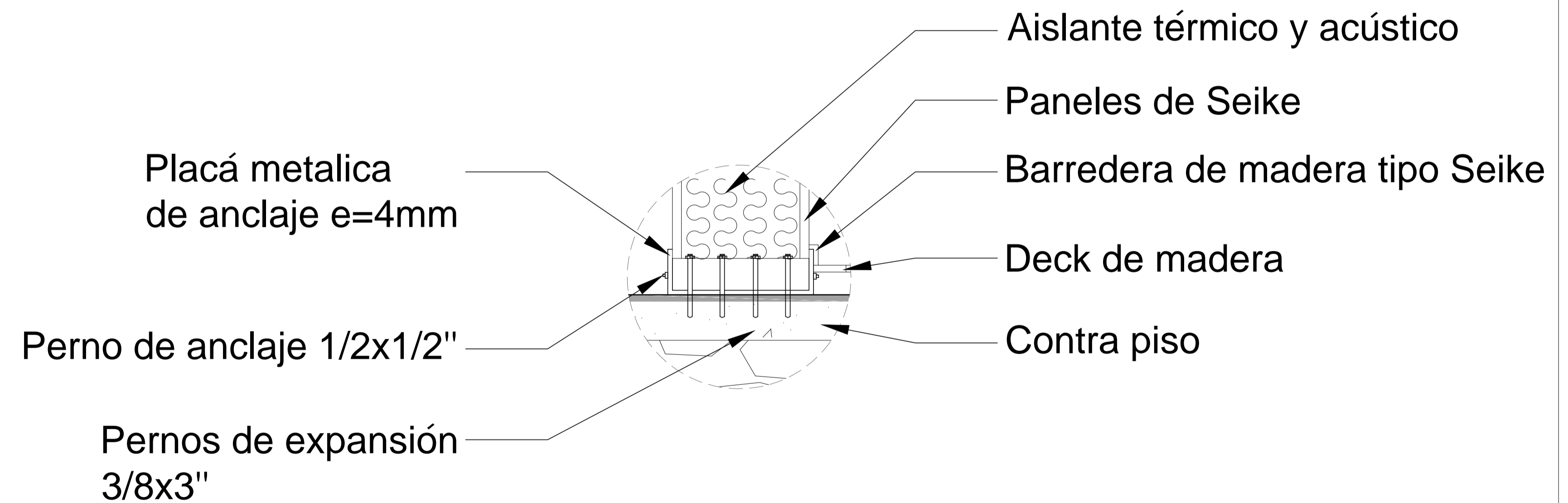
Esc 1:10 DETALLE CONSTRUCTIVO XXX
