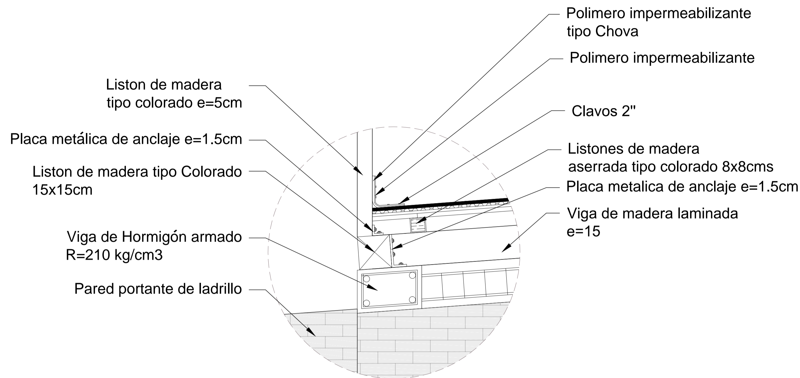
DETALLE CONSTRUCTIVO DC1 Esc 1:10
