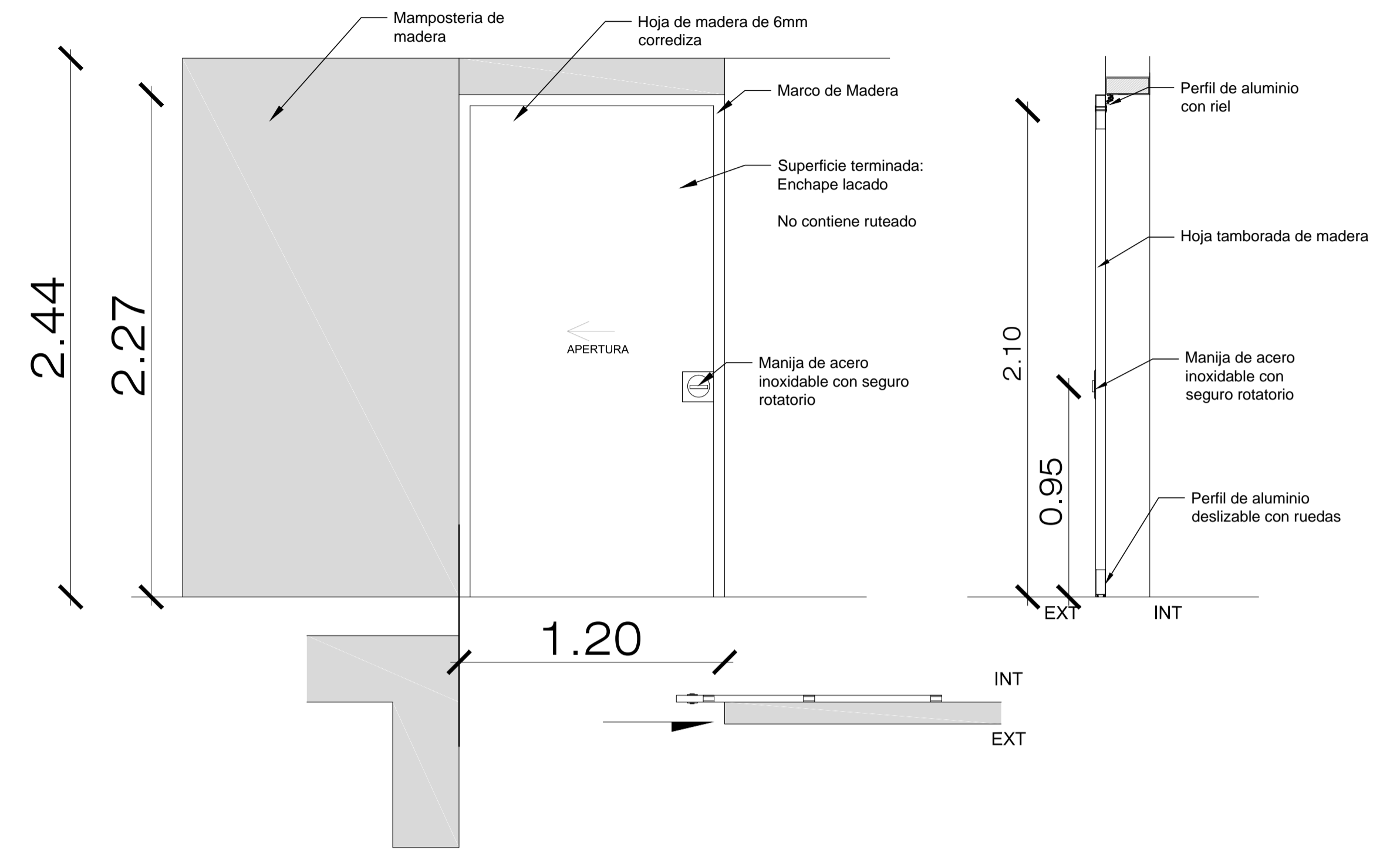
DETALLE DE PUERTA DE MADERA CORREDIZA Esc 1:20
