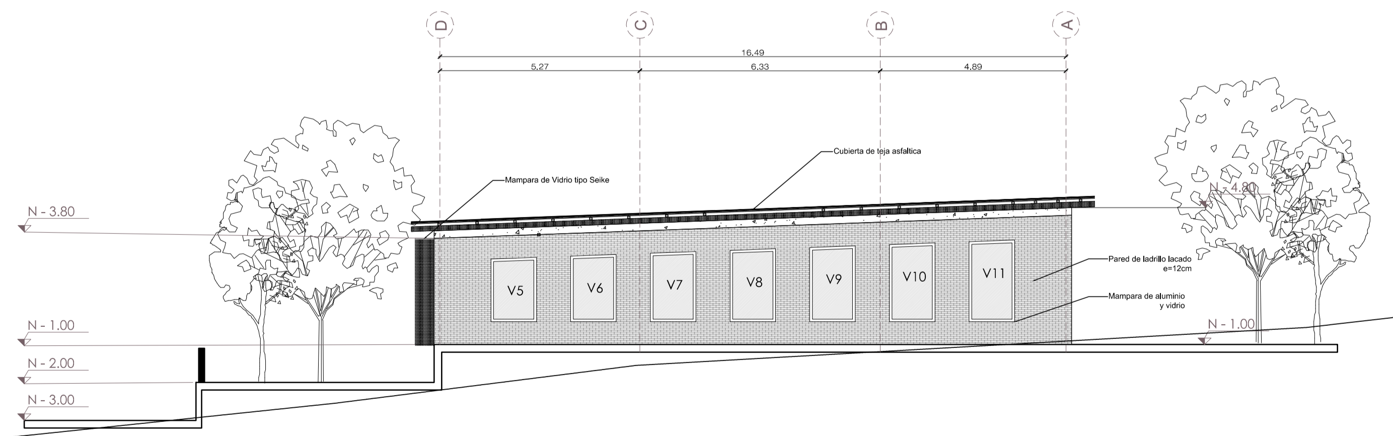
FACHADA LATERAL IZQUIERDA
