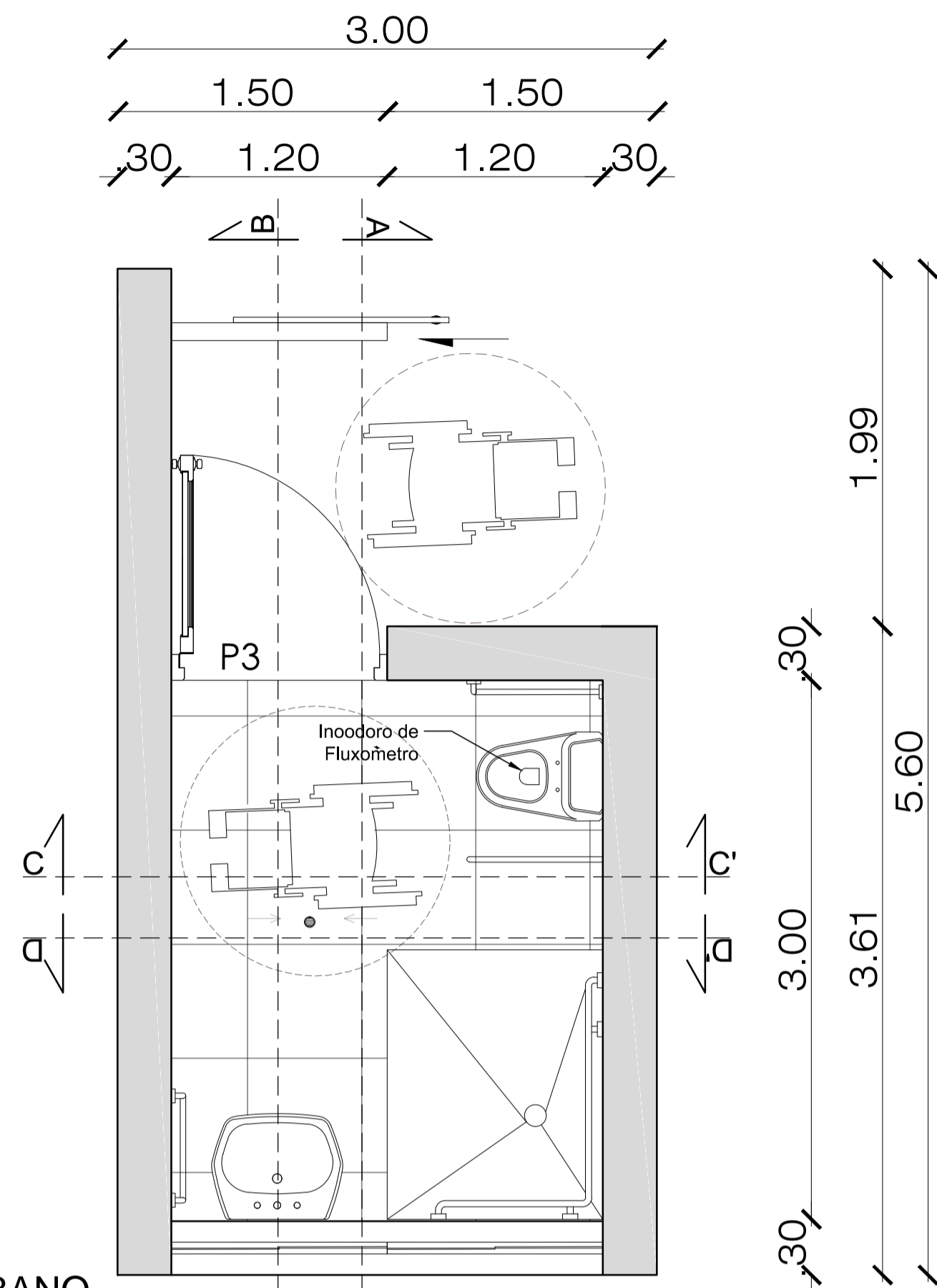
PLANTA BANO Esc 1:25
