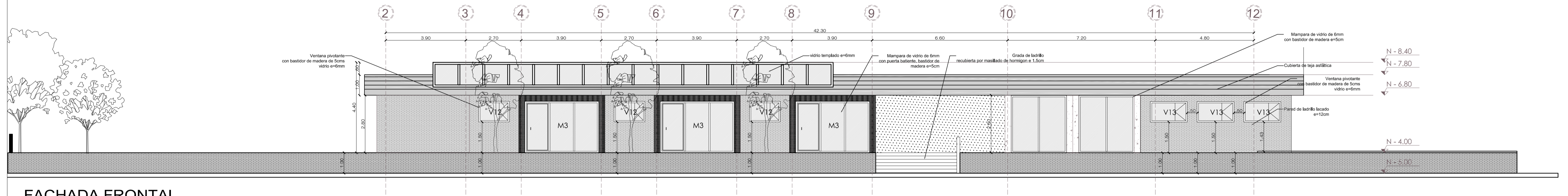
FACHADA FRONTAL
