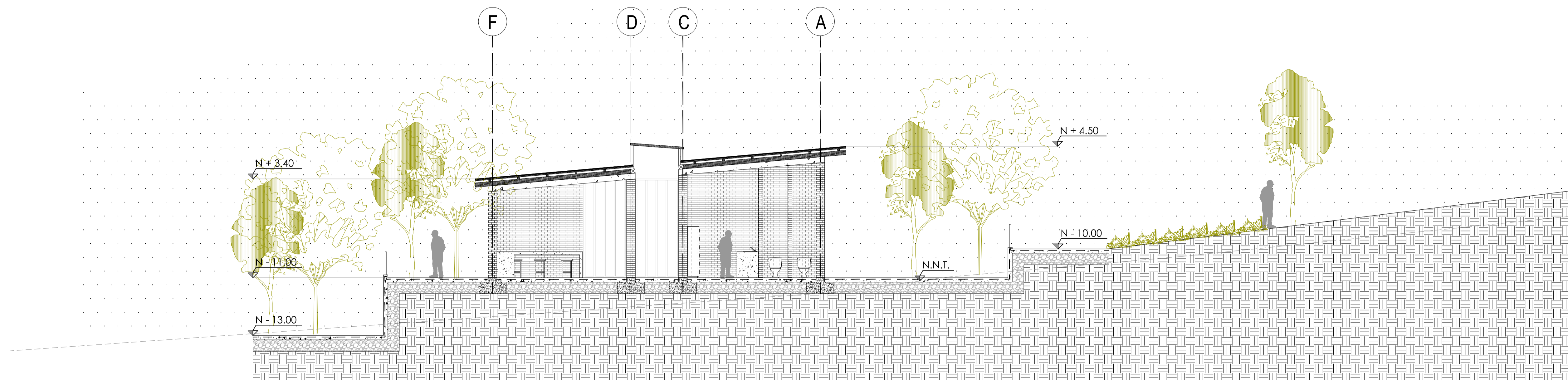
CORTE L-L'
