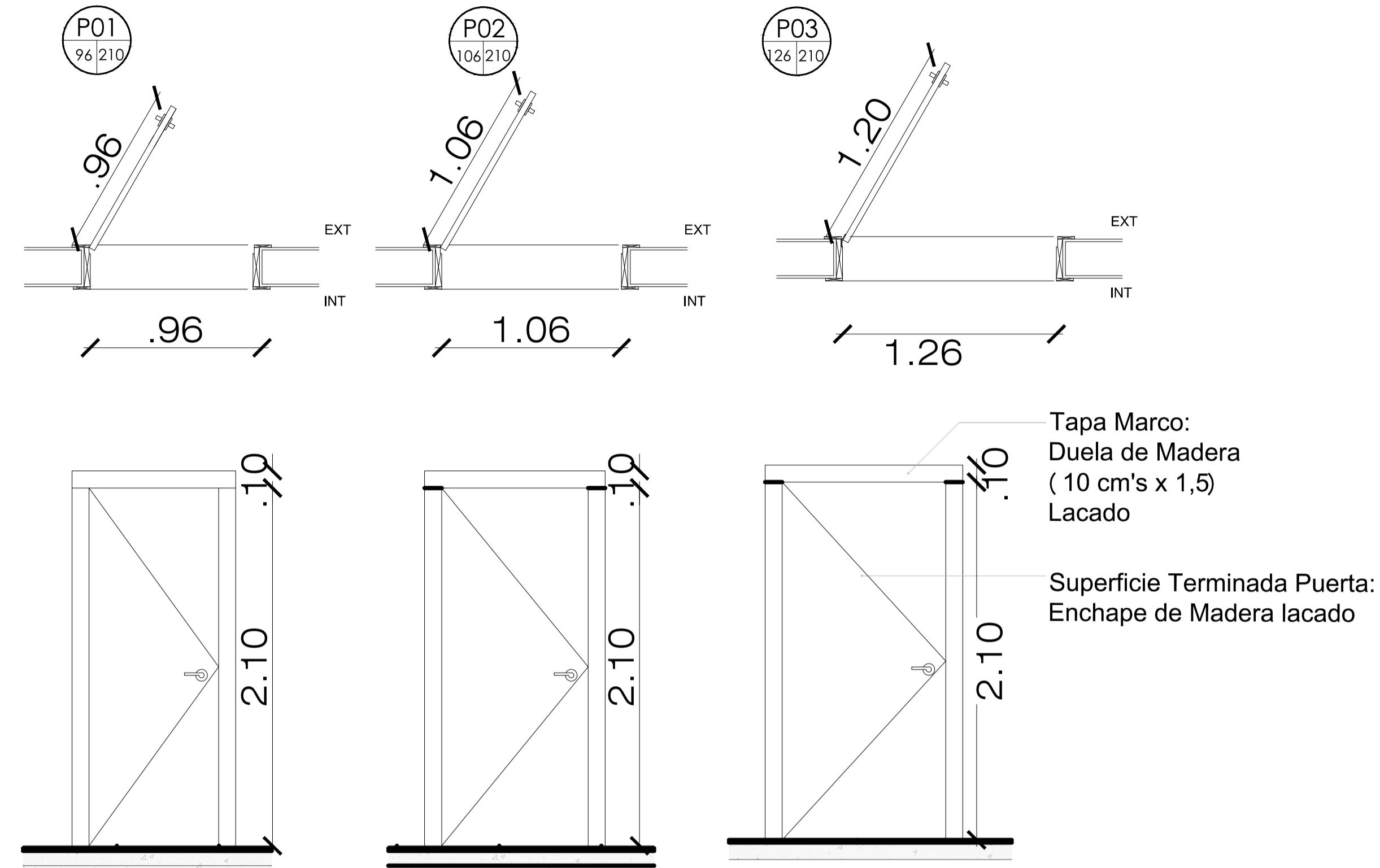
DETALLE DE PUERTAS DE MADERA Esc 1:20
