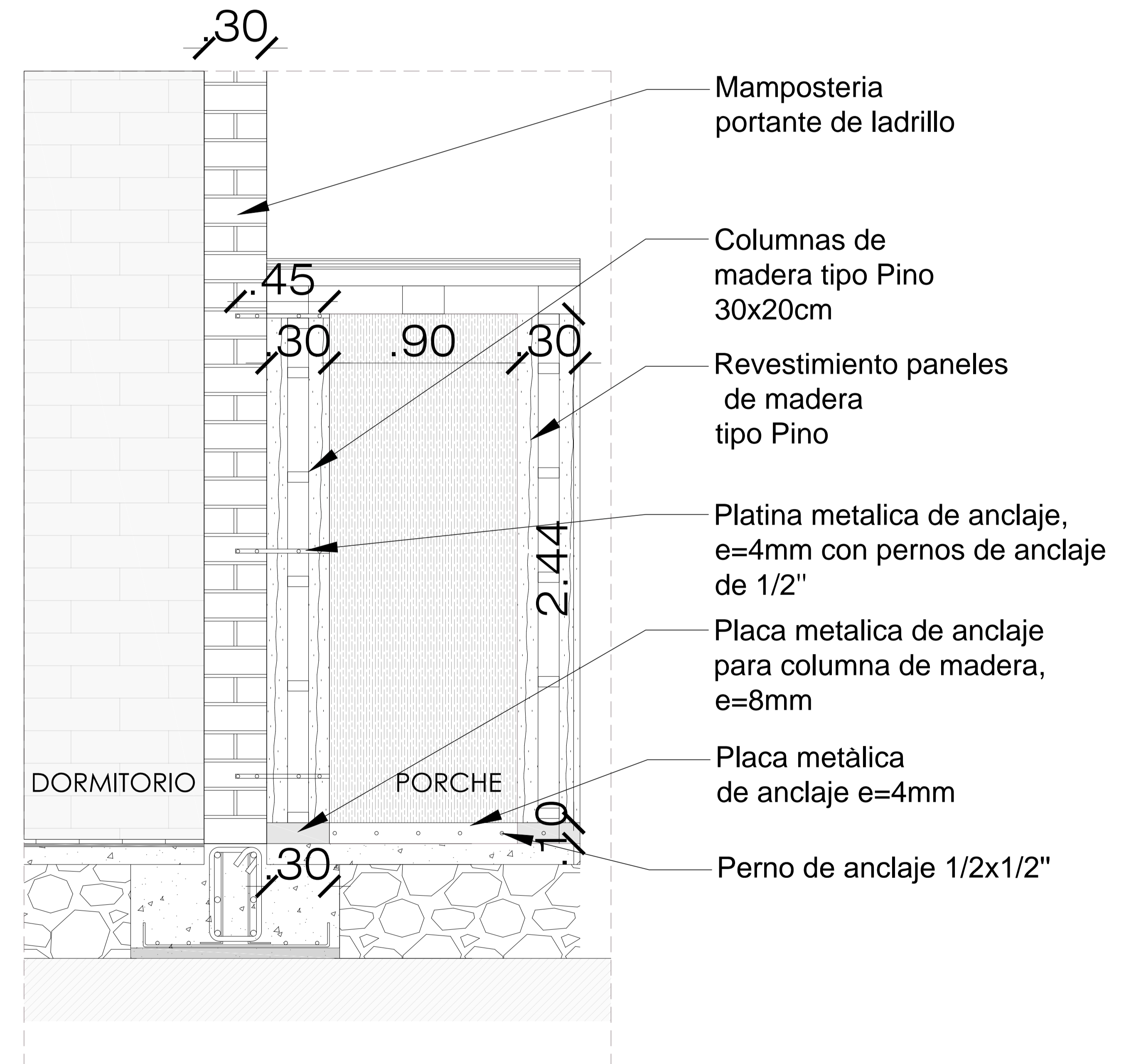
DETALLE DE JUNTA DE DORMITORIO CON CAJA DE MADERA Esc 1:15
