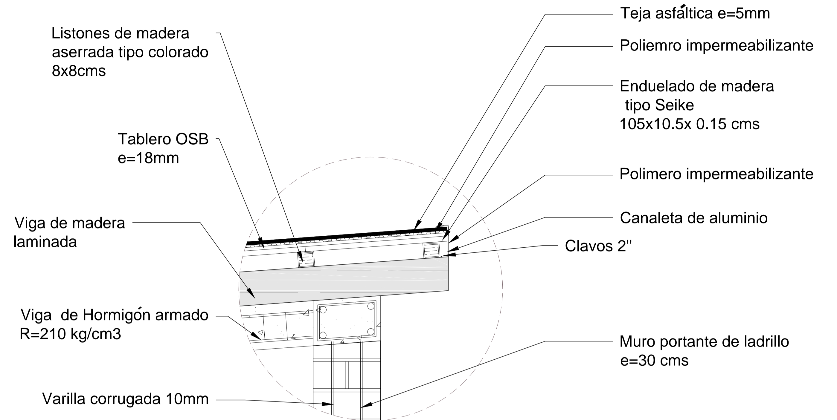
DETALLE CONSTRUCTIVO DC2 Esc 1:10
