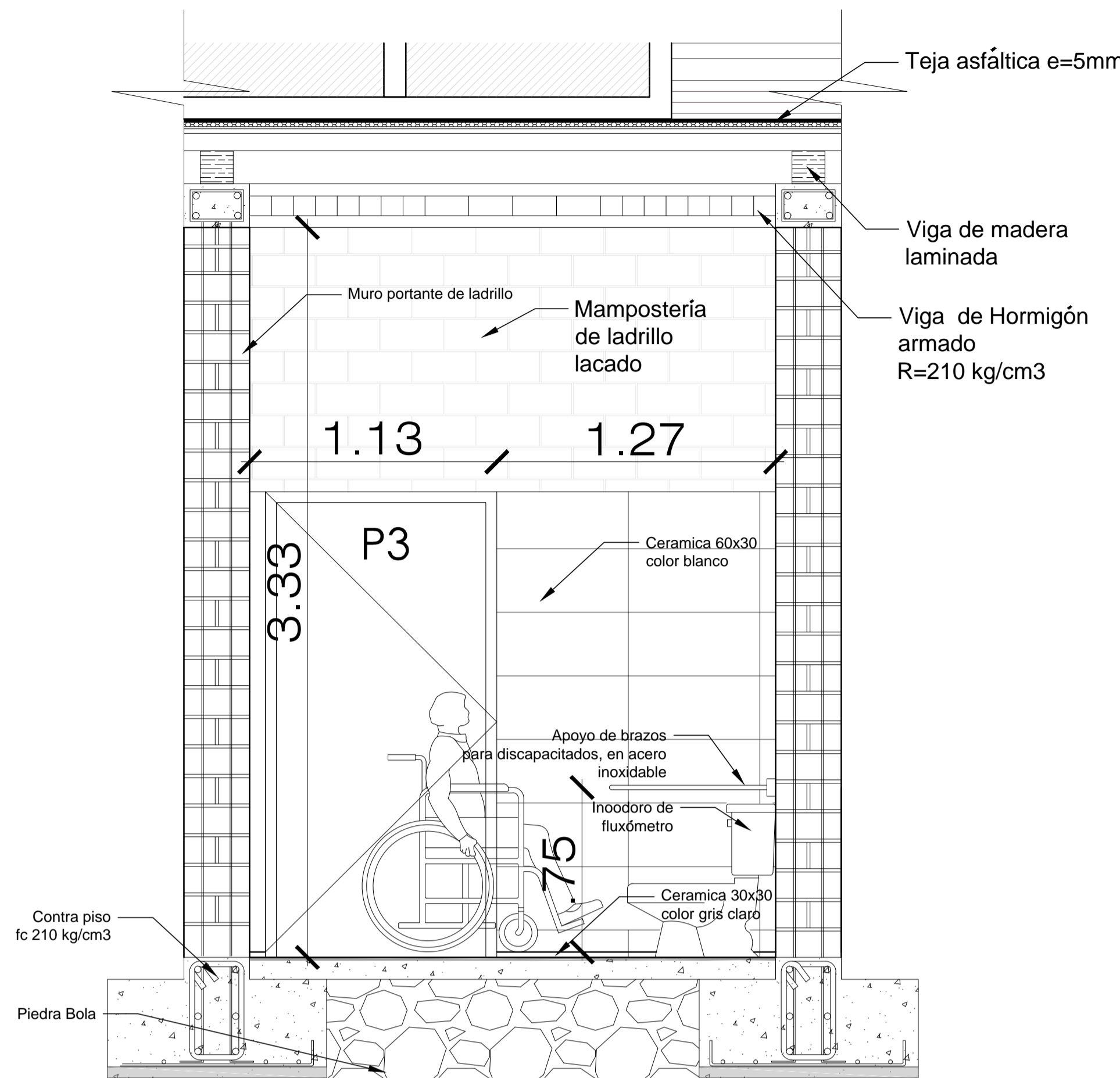
CORTE C C' Esc 1:25
