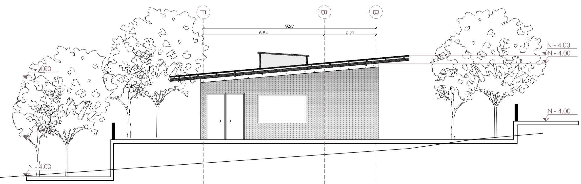
FACHADA LATERAL DERECHA
